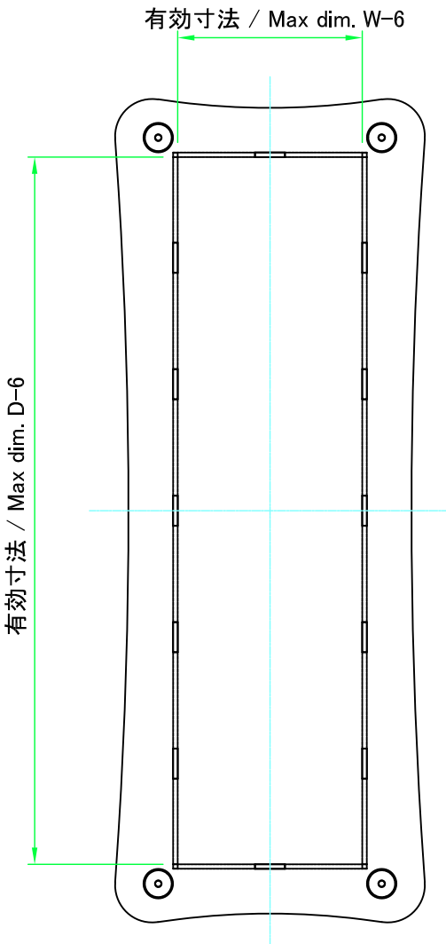
下カバー / Bottom cover
