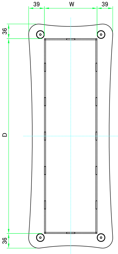
Wパネル1 / W panel 1
